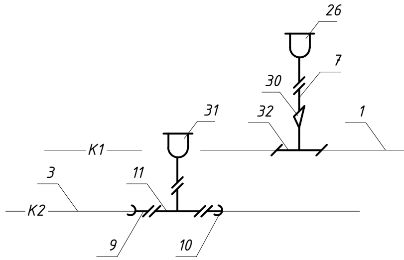
Схема колодязя 4
